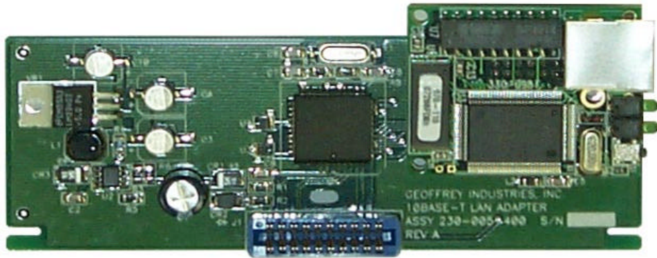
IP-Addressable Module (GIPRCNX)
