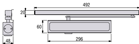
Briton 230T
